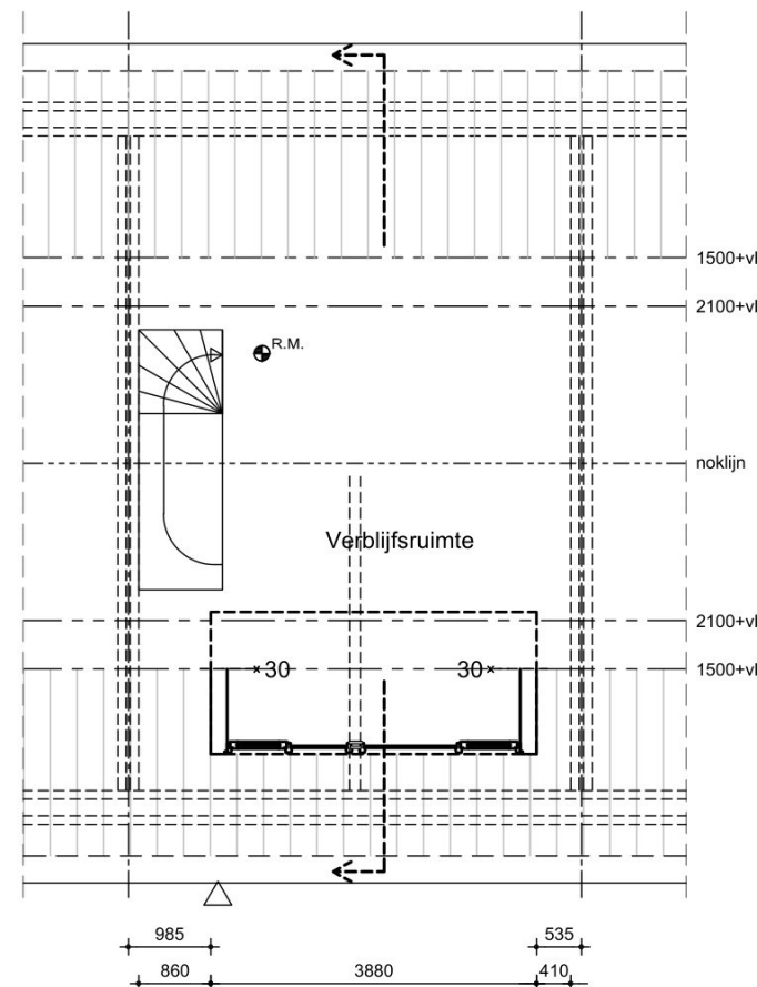
GEWIJZIGDE 2e VERDIEPING
