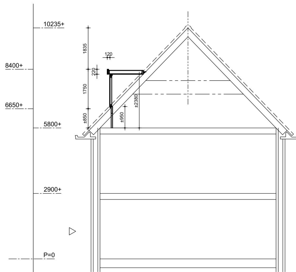
GEWIJZIGDE DOORSNEDE
