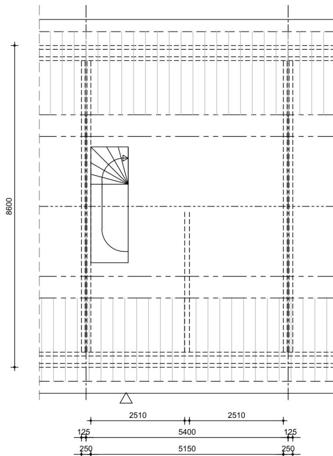
BESTAANDE 2e VERDIEPING
