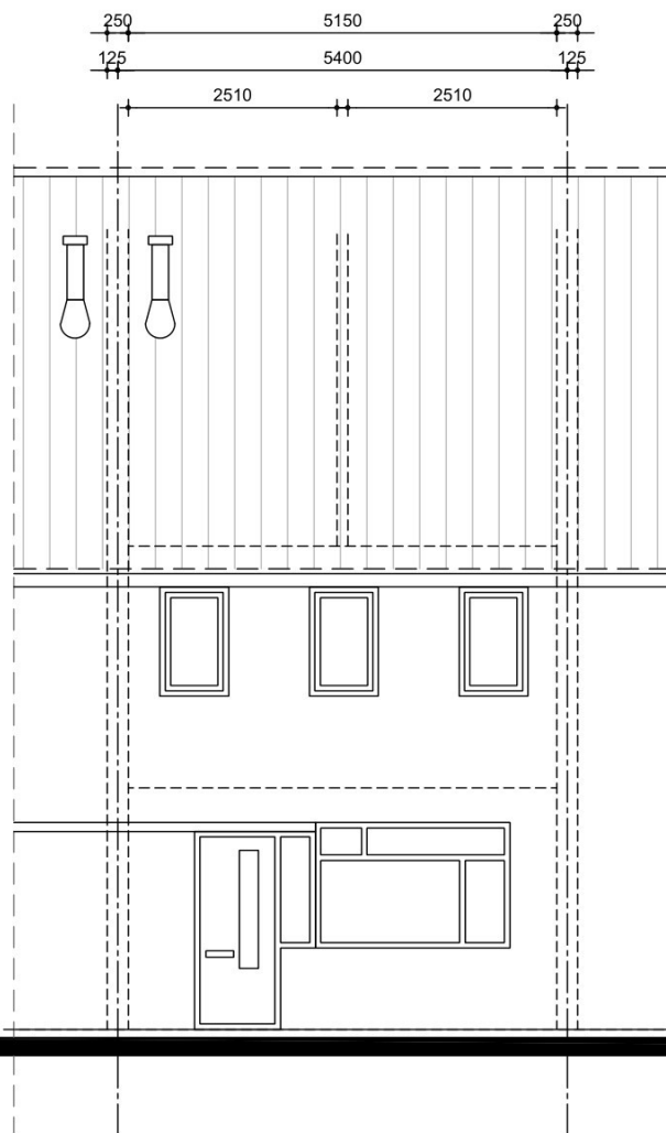
BESTAANDE VOORGEVEL
