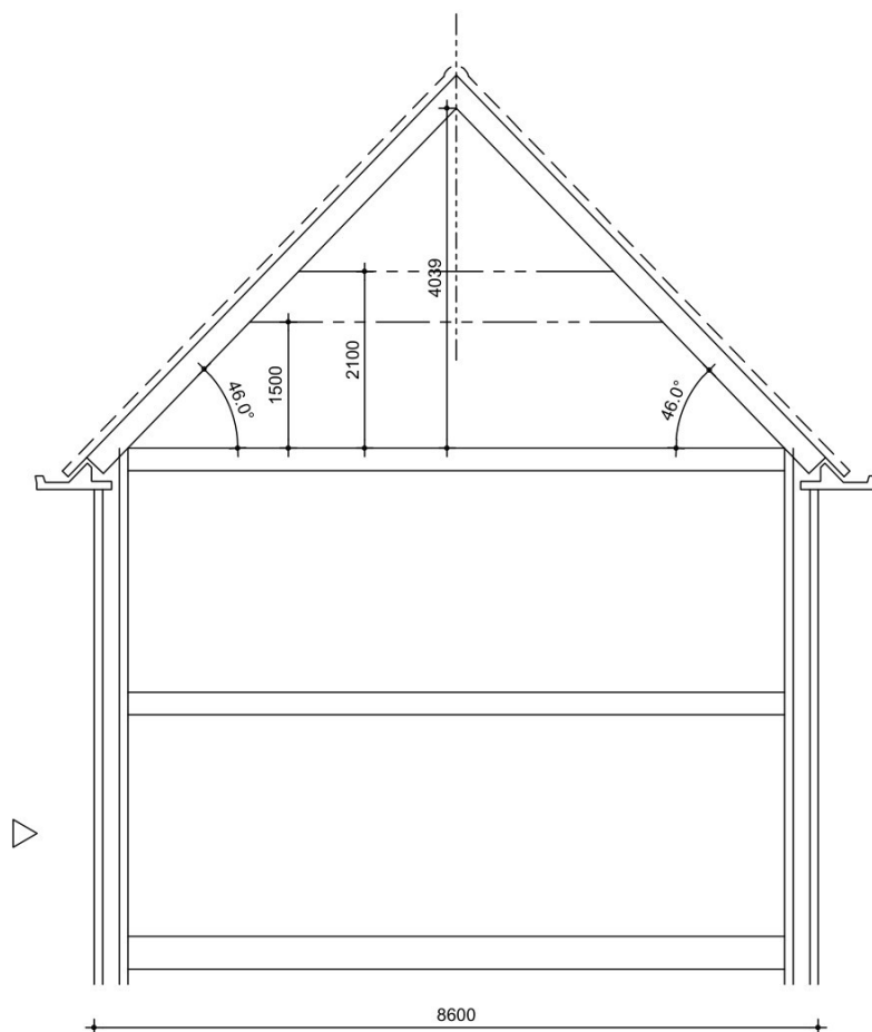
BESTAANDE DOORSNEDE
