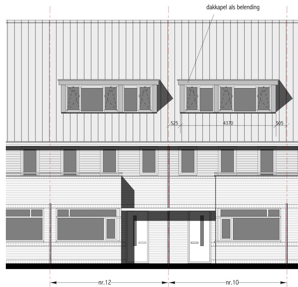
Voorgevel nieuw
