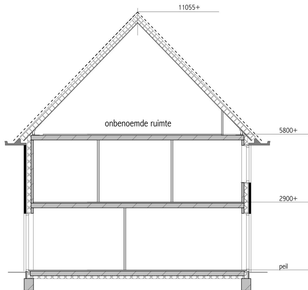
Doorsnede bestaand
