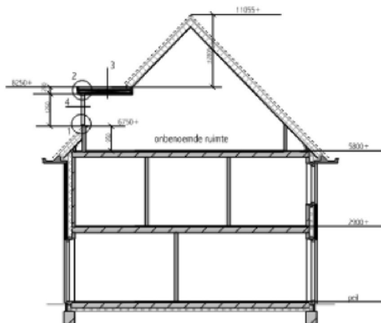
Doorsnede nieuw
