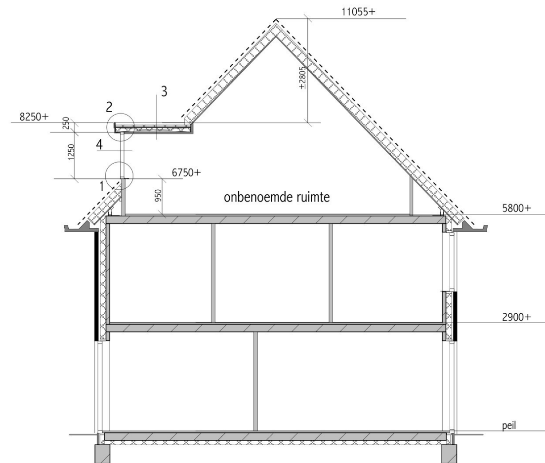
Doorsnede nieuw
