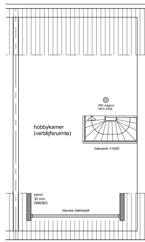
gewijzigde zolder
