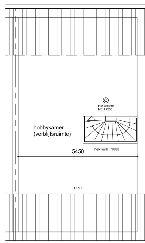
bestaande zolder
