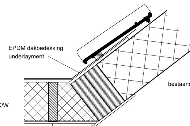
gewijzigde doorsnede
