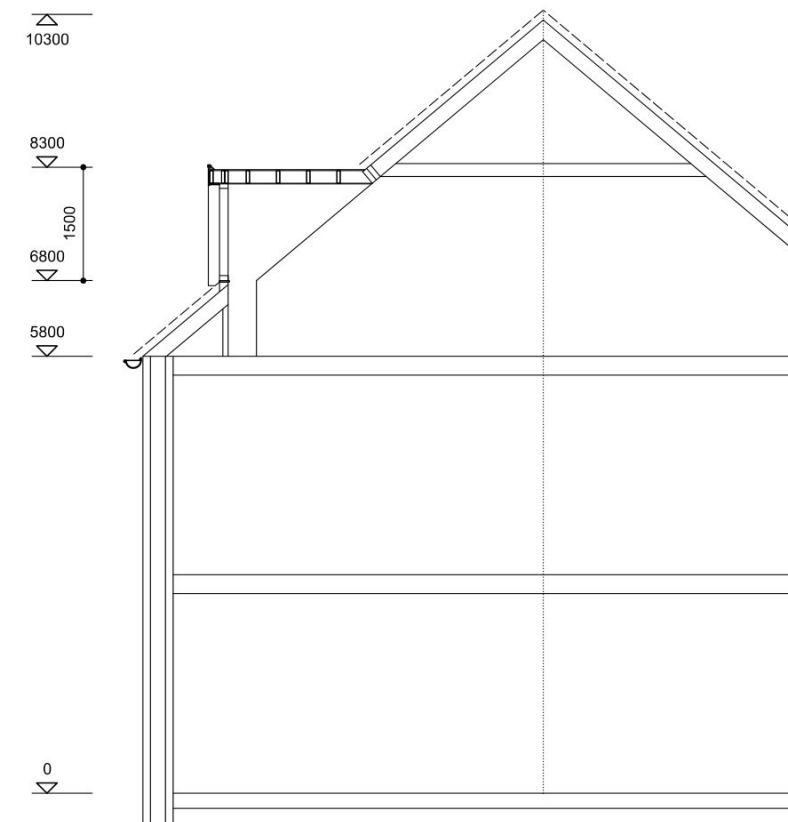
gewijzigde doorsnede
