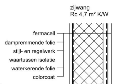
buitenzijde dakkapel uitvoeren in brandklasse D
