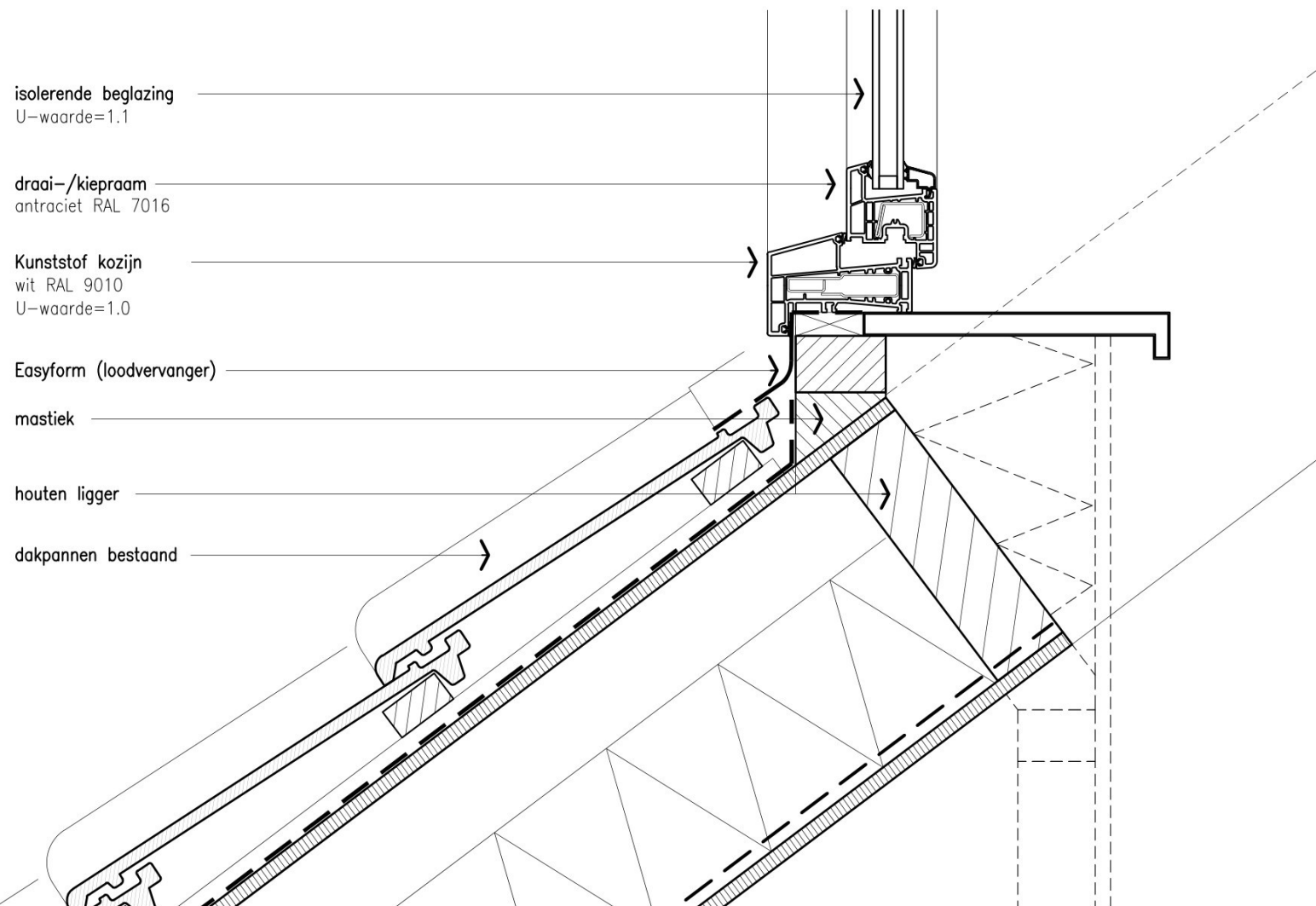
PRINCIPE DETAIL VERTICAAL V01
