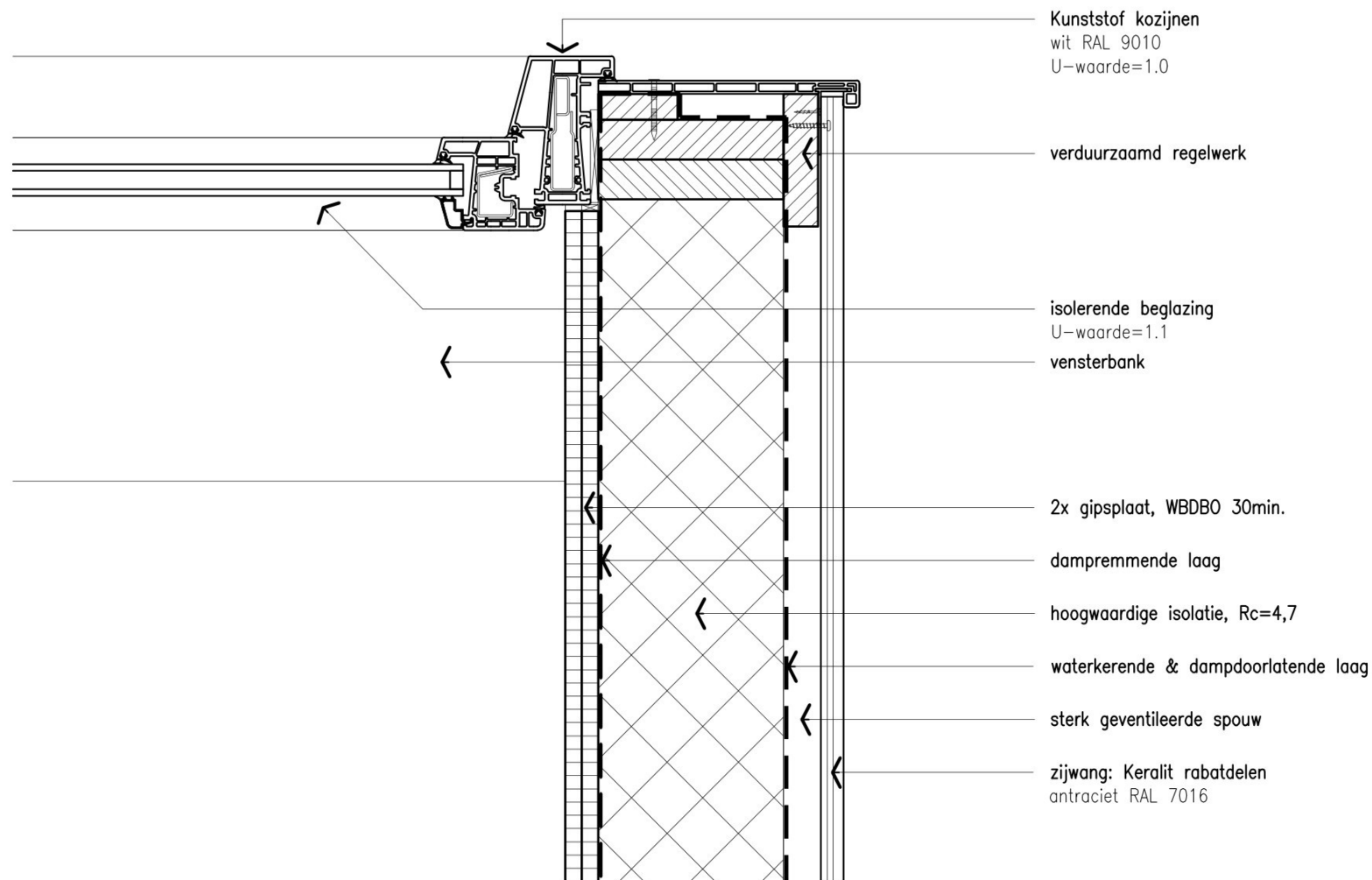
PRINCIPE DETAIL HORIZONTAAL H01
