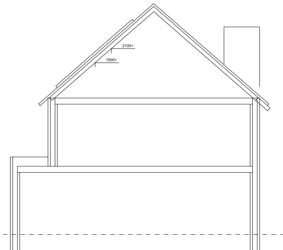
BESTAANDE DOORSNEDE
