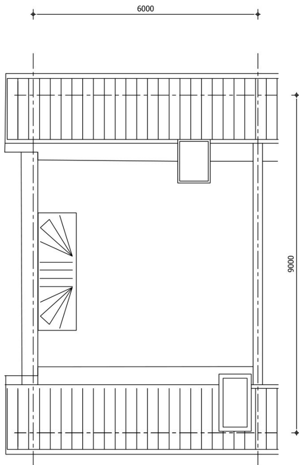
BESTAANDE 2e VERDIEPING
