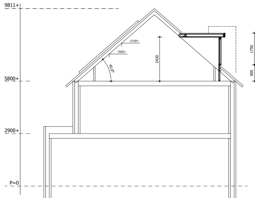
GEWIJZIGDE DOORSNEDE
