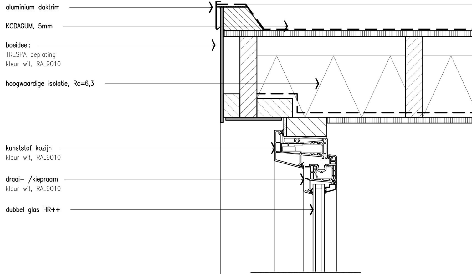
PRINCIPE DETAIL VERTICAAL V02
