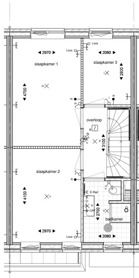
Eerste verdieping
