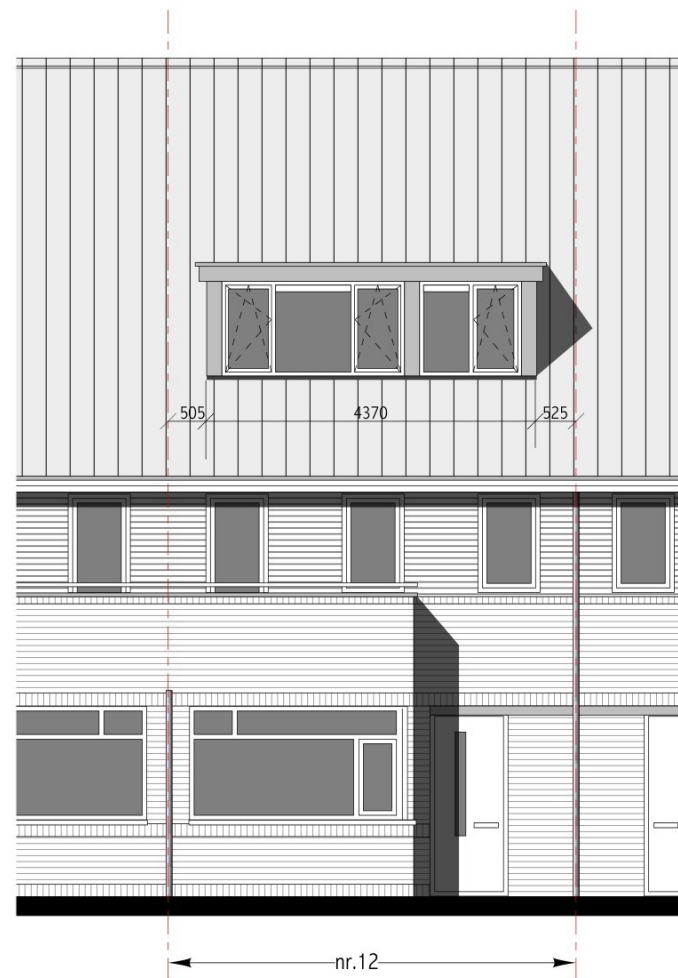
Voorgevel nieuw
