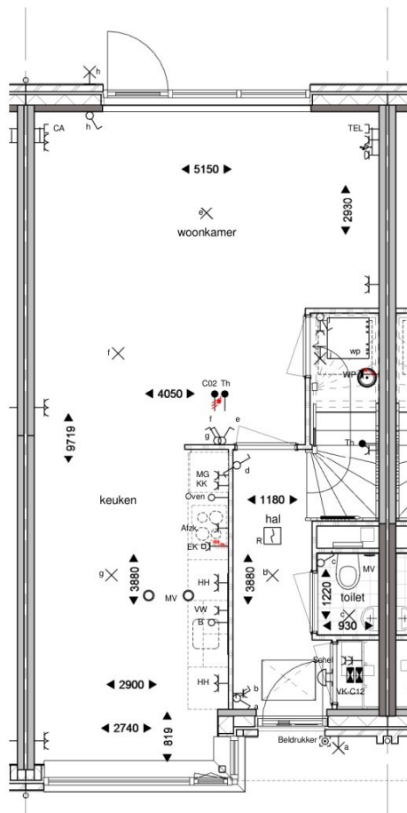
Begane grond
