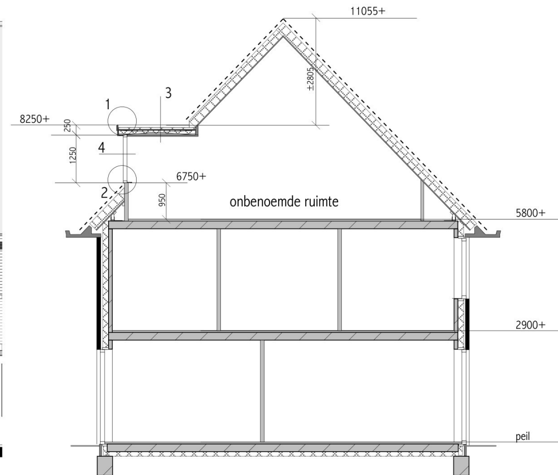
Doorsnede nieuw
