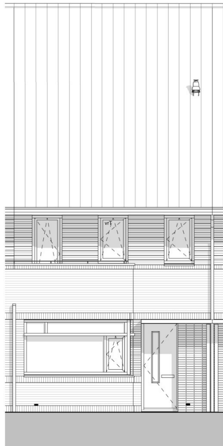
Vorgevel
