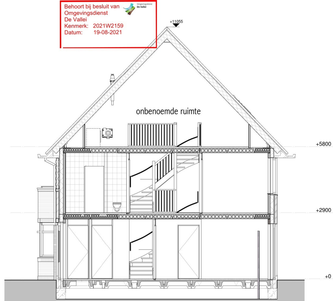
Doorsnede
