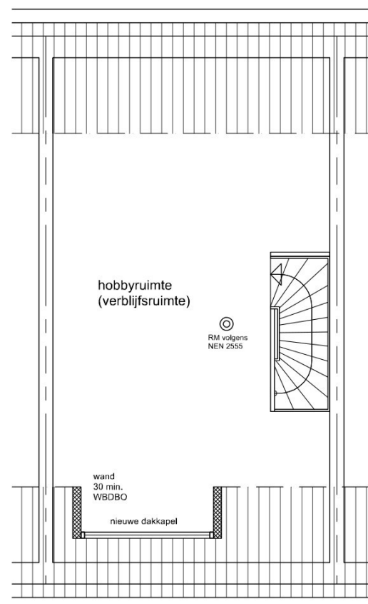
gewijzigde zolder
