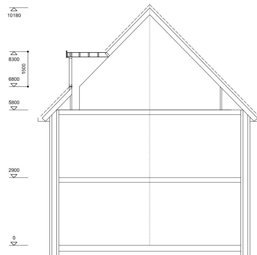
gewijzigde doorsnede
