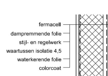
bestaande doorsnede
